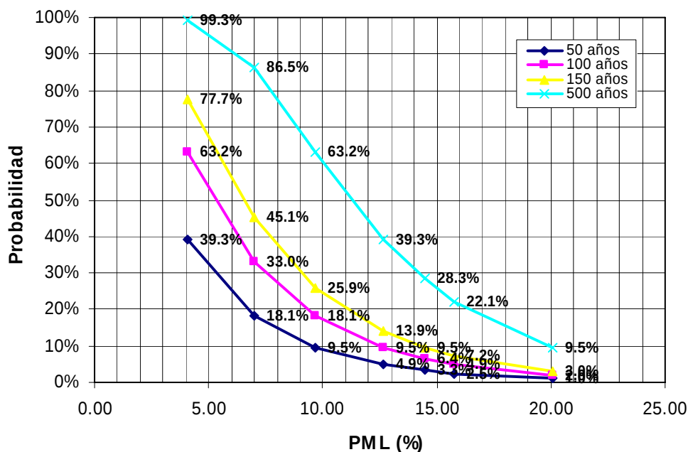
Figura 2.3 Curva de PML para diferentes tiempos de exposición y probabilidades de excedencia
