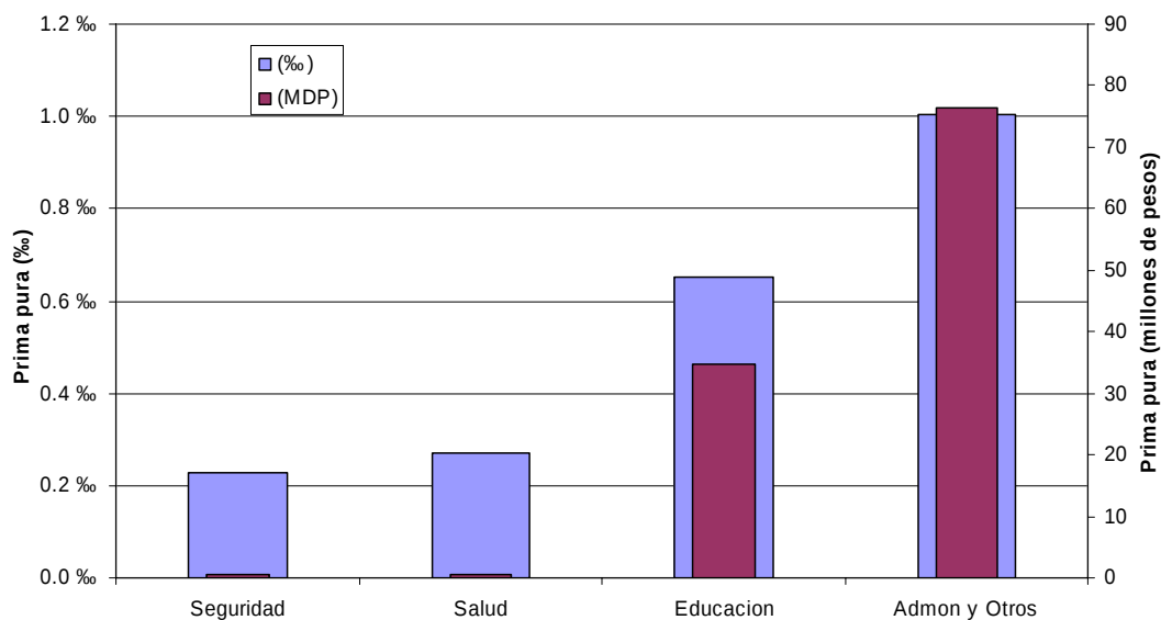
Figura 2.18 Comparación de PML 1500 entre sectores
