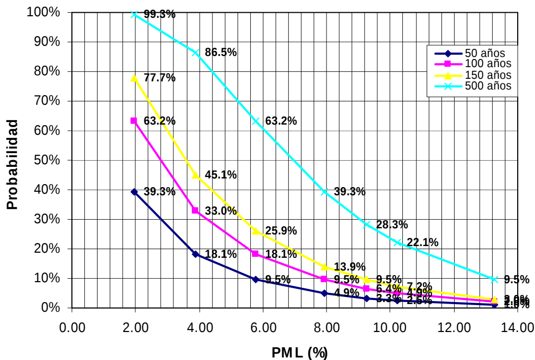
Figura 2.12 Curva de PML para diferentes tiempos de exposición y probabilidades de excedencia
