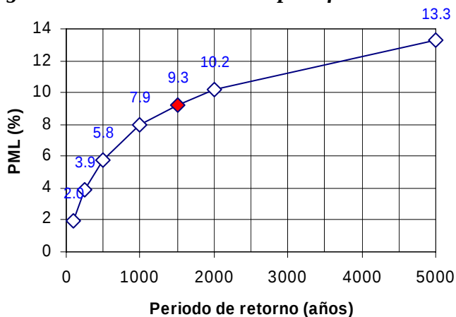
Figura 2.11 Curva de PML del portafolio intervenido
