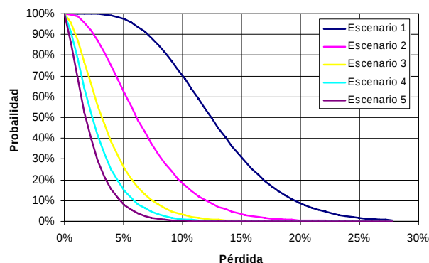
Figura 2.14 Probabilidad de quiebra para los escenarios sísmicos más desfavorables
