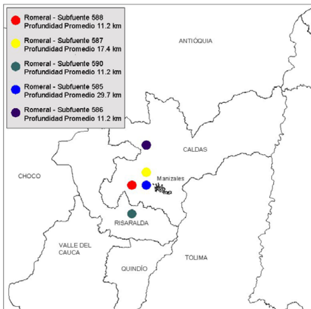
Figura 2.4 Ubicación de los escenarios sísmicos más desfavorables
